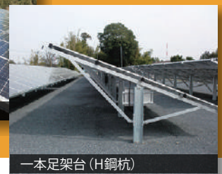
一本足架台(H鋼杭)
